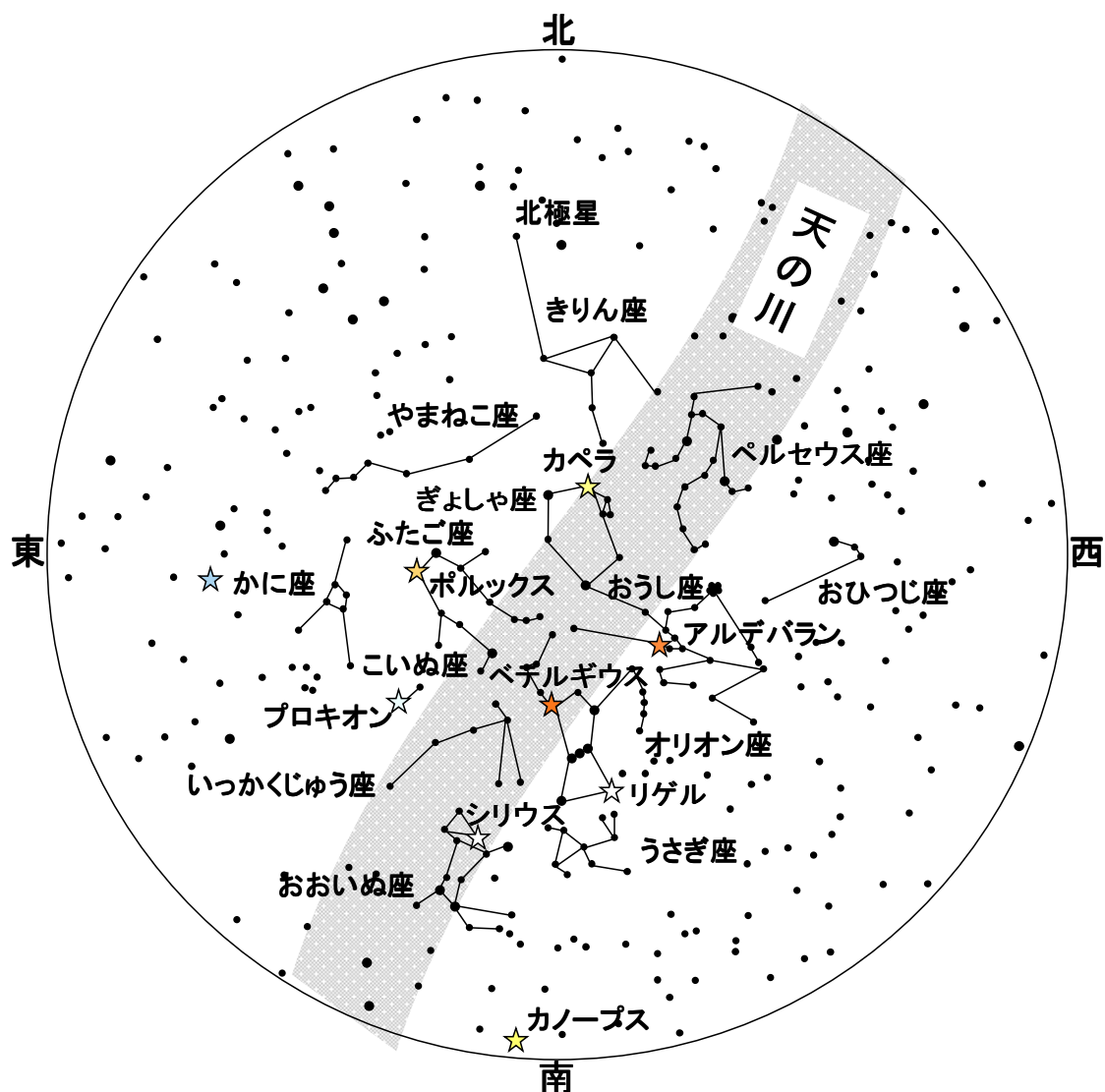
図 2-8 冬の星座たち
