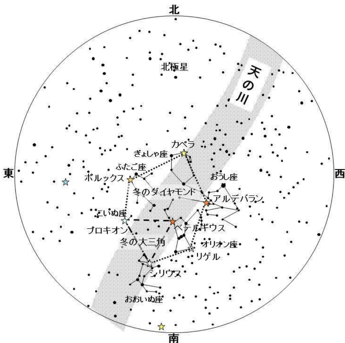
図 2-9 冬の星座の見つけ方
